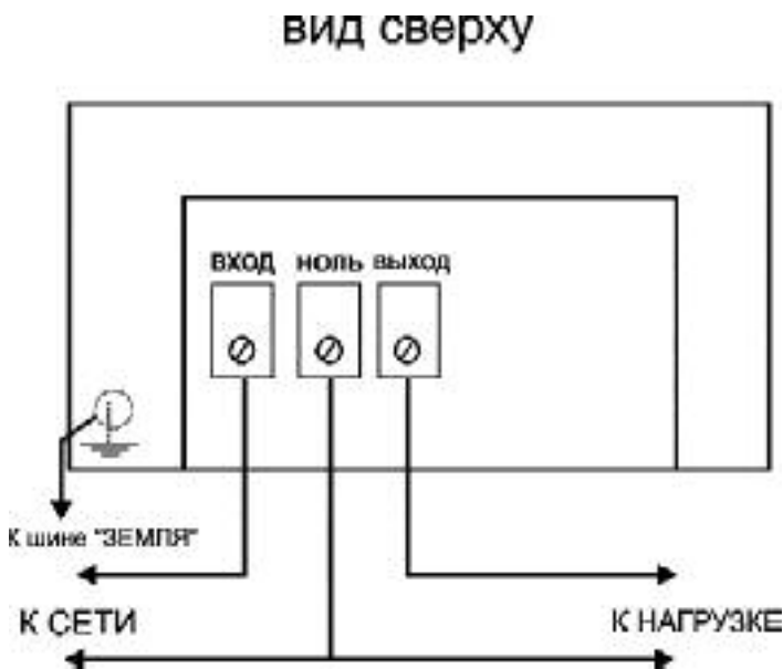
Рис.3. Подключение стабилизатора к сети и к нагрузке
